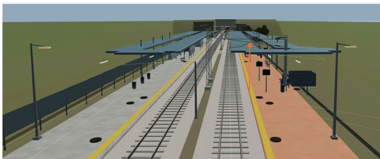
Prostorový model s vybraným nástupištěm.
